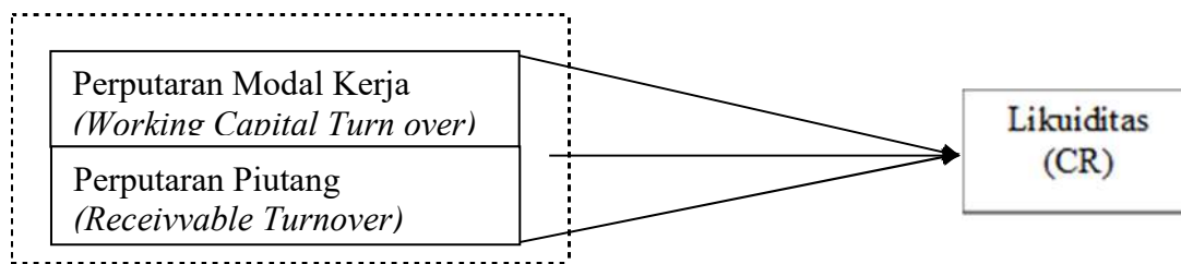
Gambar 1. Kerangka Fikir
